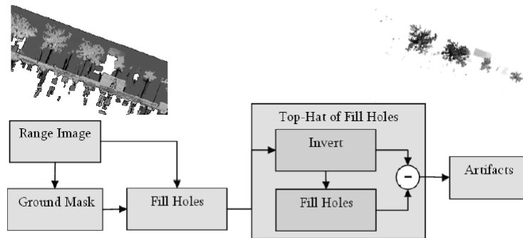
Rys. 3.1. Algorytm wykrywania obiektów (Hernández i Marcotegui, 2009b)
