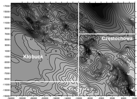
Rys. 4. Cyfrowy model geomorfologiczny podłoża czwartorzędu z wydzielonymi podobszarami badawczymi Kłobuck i Częstochowa
