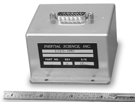
Fig. 3. ISIS-IMU
