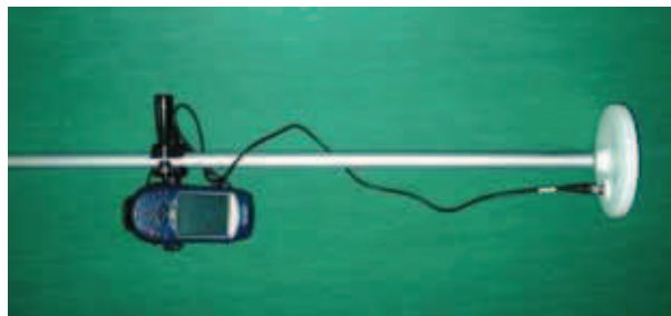
Rys. 2. Mobile Mapper CX z anteną zewnętrzną
