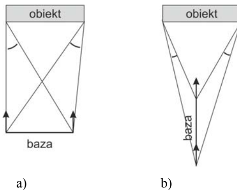
Rys. 3. Warunki wycięcia w przód dla dwóch różnych konfiguracji osi kamery względem linii bazy; a) baza prostopadła, b) baza równoległa do osi obserwacyjnej
