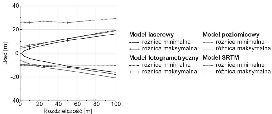
Rys. 3. Ekstremalne błędy wysokości w poszczególnych modelach terenu
