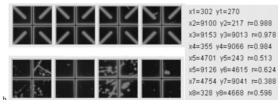
Rys. 1. Automatyczny pomiar współrzędnych znaczków tłowych
