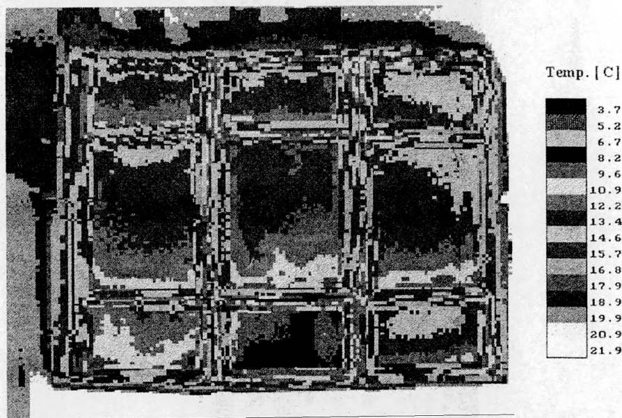
Rys. 4.: Zmontowany termogram okna (infiltracja zimnego powietrza do wnętrza pomieszczenia: a) nieszczelności pomiędzy ramą a ościeżnicą okna; b) wybita jedna szyba (okna były dwu szybowe)
